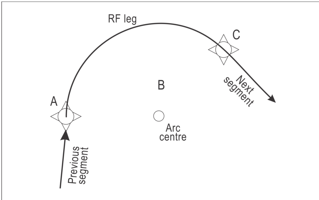
Figure II-1-1-4. RF turn
